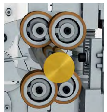
Zentrierlünette zwischen Führungskanal und Spindeleinsatzrohr
